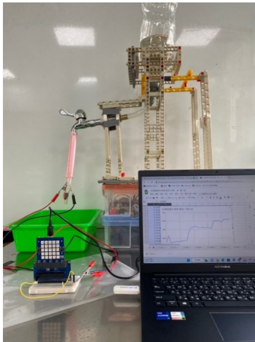
圖 10：水龍頭漏水實測實驗模組圖(側面)
