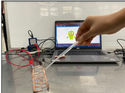
圖 7：模擬漏水實驗- 銅箔 (砂紙塑膠片)
