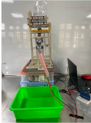
圖 11：水龍頭漏水實測實驗模組圖(正面)
