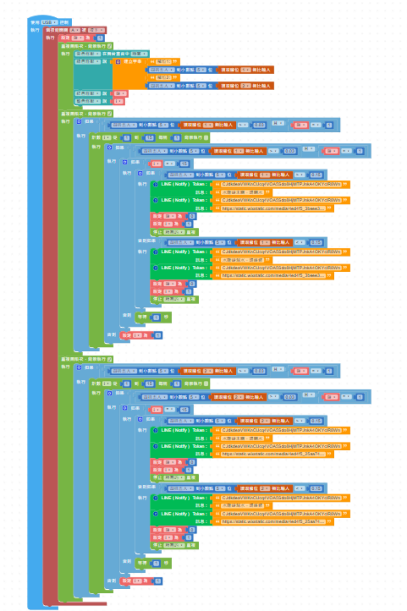
圖 33: 銀箔磨砂間距中及 LINE 即時回報系統程式圖
