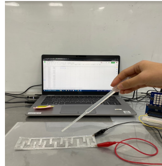
圖 8：模擬漏水實驗- 銀箔 (砂紙塑膠片)
