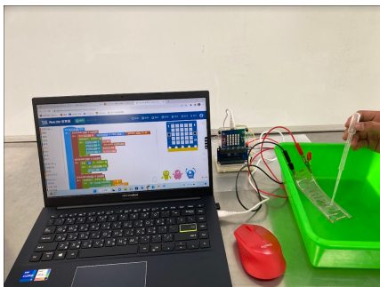
圖 9：模擬漏水實驗- 銀膠 (砂紙塑膠片)
