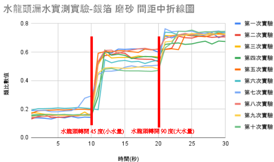
圖 29：水龍頭漏水實測實驗-銀箔磨砂間距中(間隔 0.5cm) 折線圖
